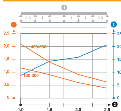
Belastningsdiagram kabelbakke type RKS-Magic 60
